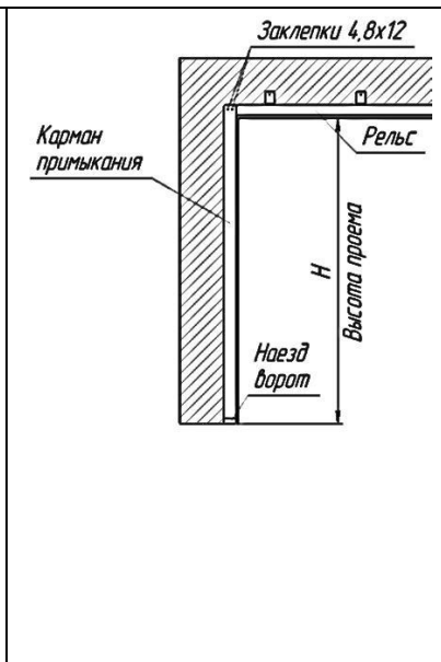
8. Монтаж наезда ворот и кармана примыкания
