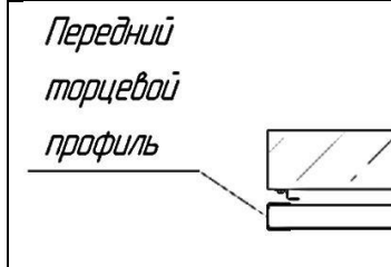
14. Установка переднего торцевого профиля
