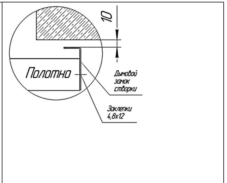
9. Установка дымового замка створки
