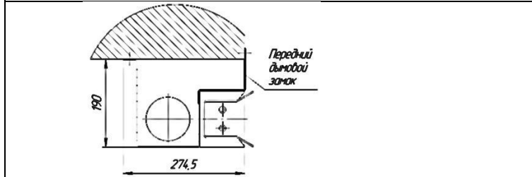
16. Установка переднего дымового замка
