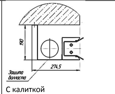
10. Установка настенного дымового замка
