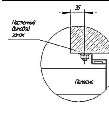
10. Установка настенного дымового замка
