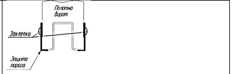
15. Защита порога
