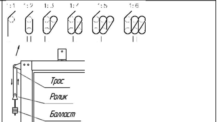
11. Установка балласта
